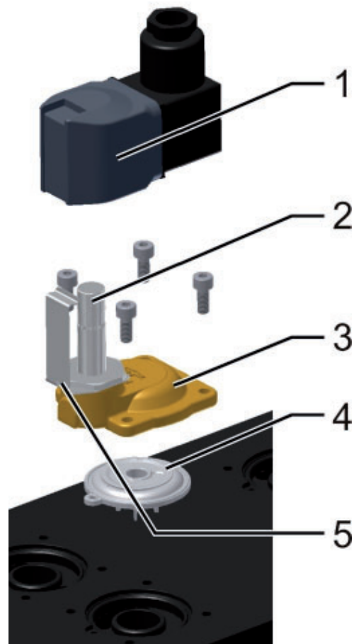
Magneetventiel
