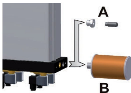
Geluiddemper losdraaien
